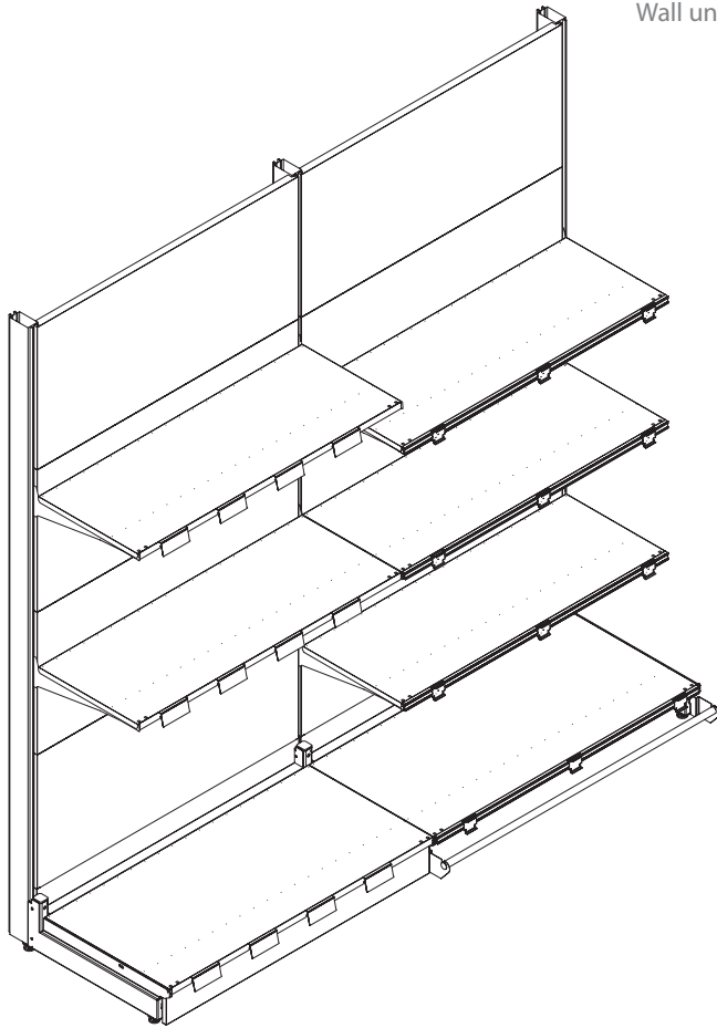
Elemento a gondola con piani ExtraSlim e Mini-ExtraSlim ExtraSlim and Mini-ExtraSlim gondola unit
