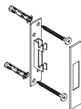
Fissaggio diretto a parete con supporto per fissaggio, carter di chiusura, viti e tassello Direct fixing with support and cover for wall
